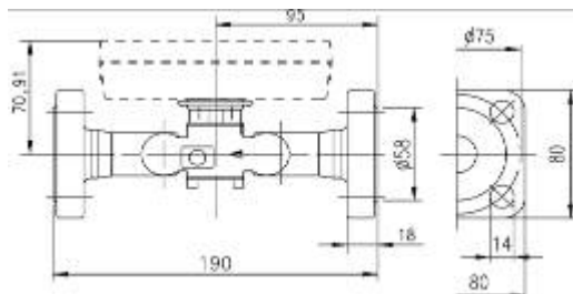
Установочная длина 190 мм (фланцевое исполнение)
